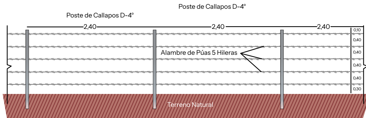
Figura 38. Cerco perimetral con alambre de púas.
