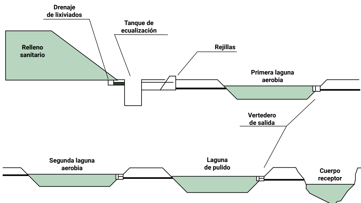
Figura 24. Lagunas de Estabilización
