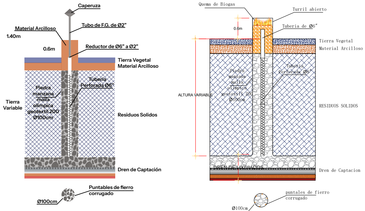
Figura 25. Construcción referencial de chimeneas.
