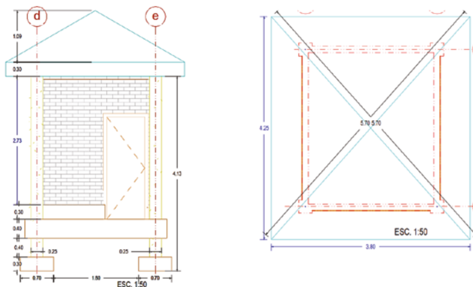
Figura 39. Vista frontal y en planta – Caseta de control
