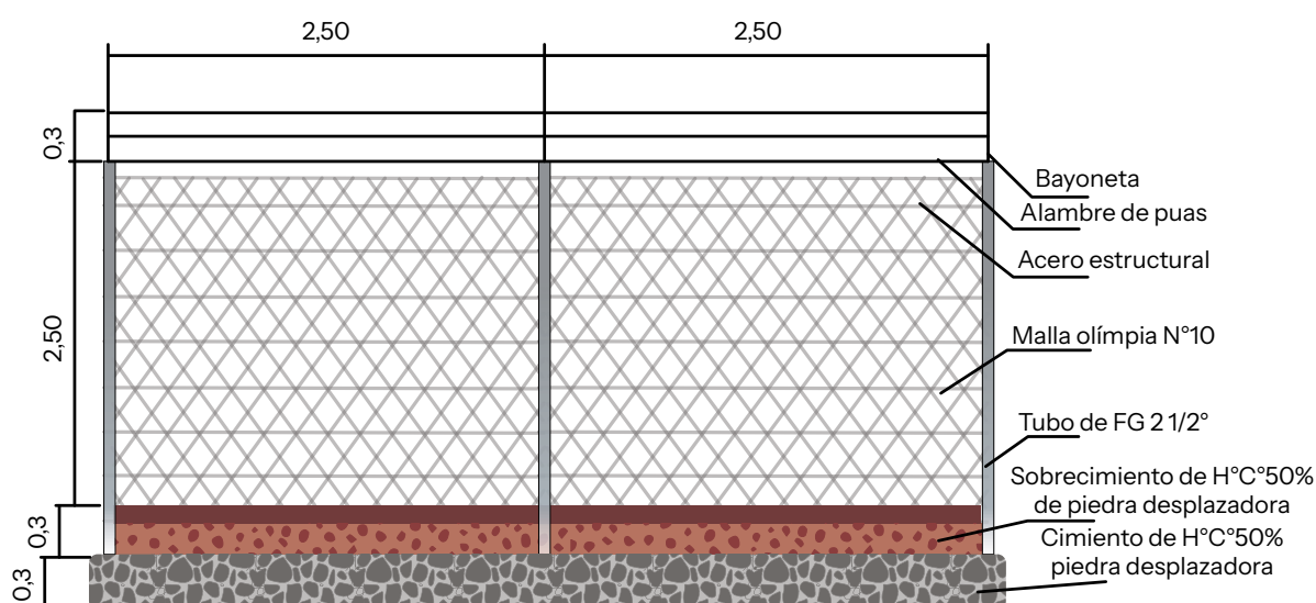
Figura 37. Cerco perimetral con malla olímpica.
