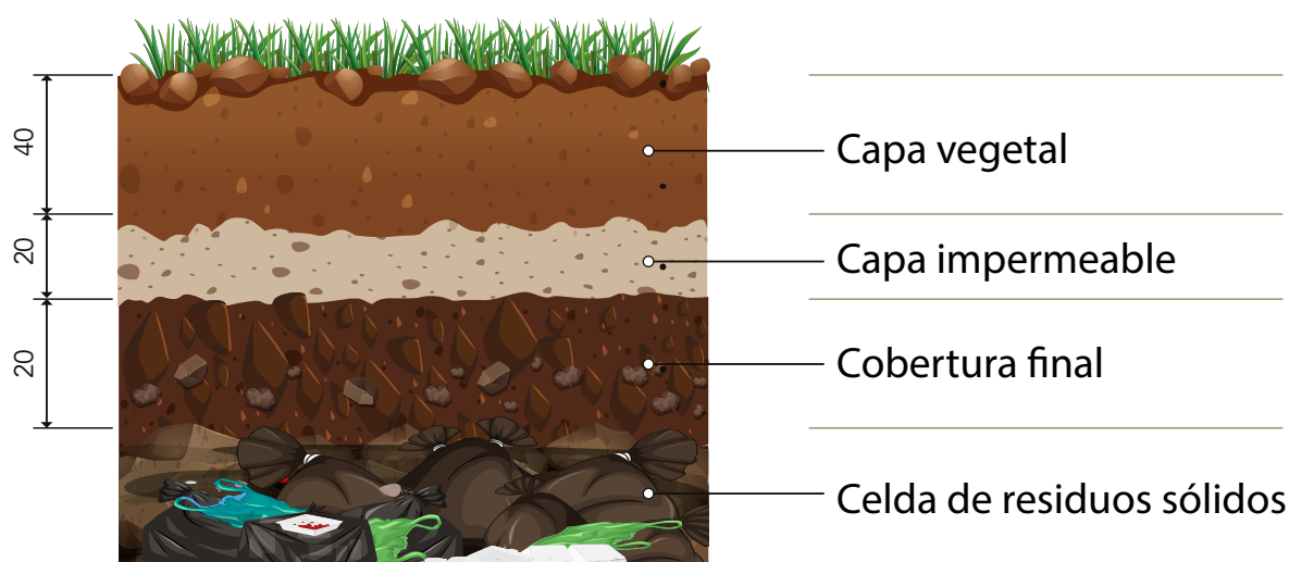
Figura 60. Capa final de la celda.
