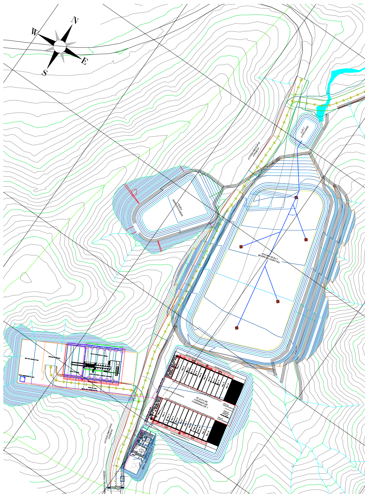
Figura 8. Planimetría del Complejo de Tratamiento de Residuos de Camiri.
