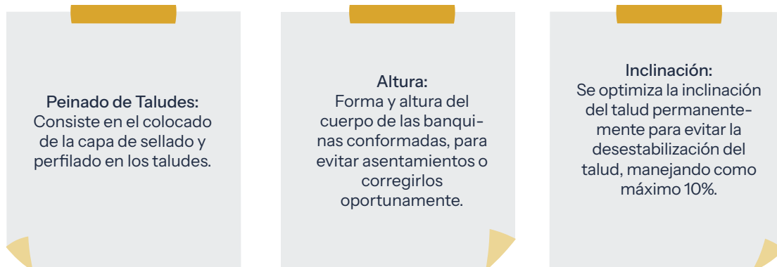
Figura 48. Recomendaciones en un crecimiento vertical de celdas.
