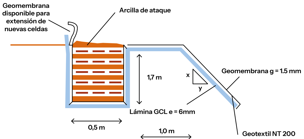
Figura 36. Anclaje geomembrana.
