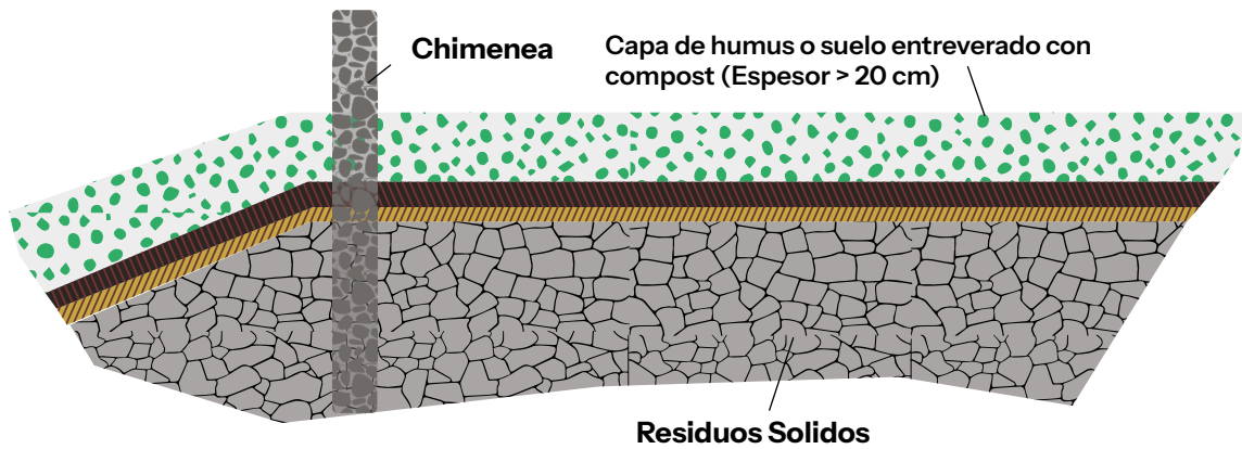
Figura 62. Aplicación de capa de humus.
