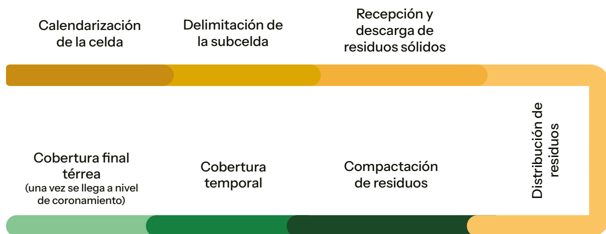
Figura 43. Los 8 pasos en la operación de celdas de un relleno sanitario semimecanizado.
