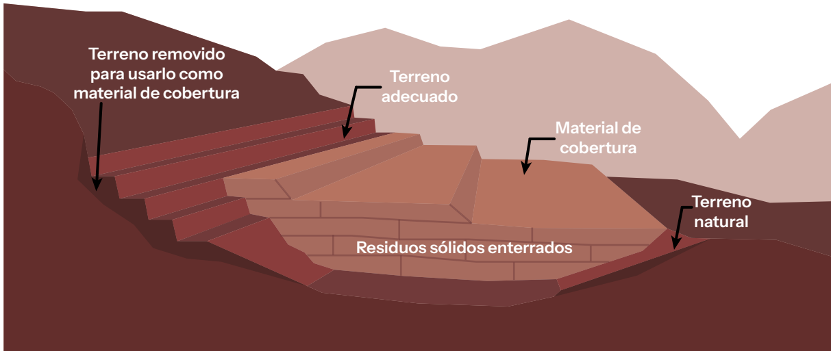
Figura 12. Método combinado (área y trinchera).
