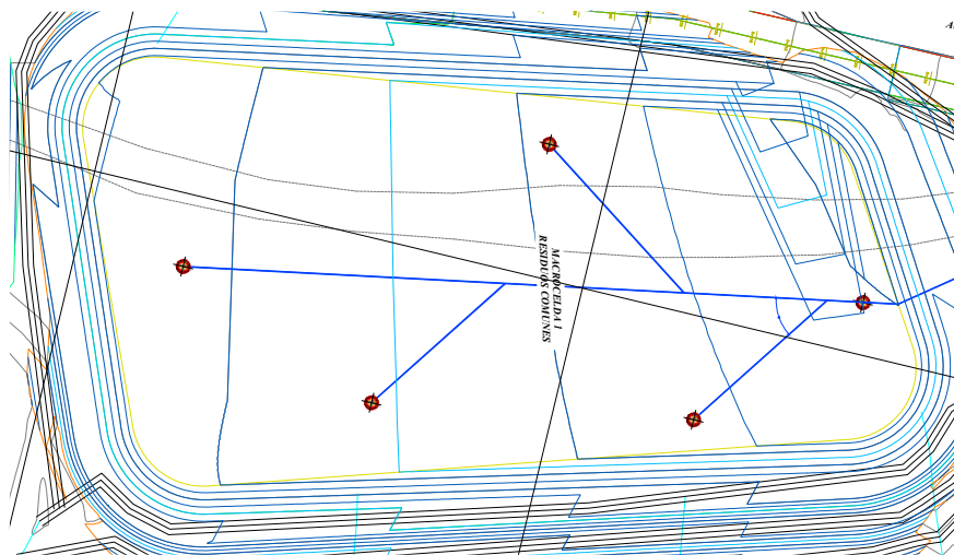
Figura 21. Distribución de sistema de drenaje de lixiviados
