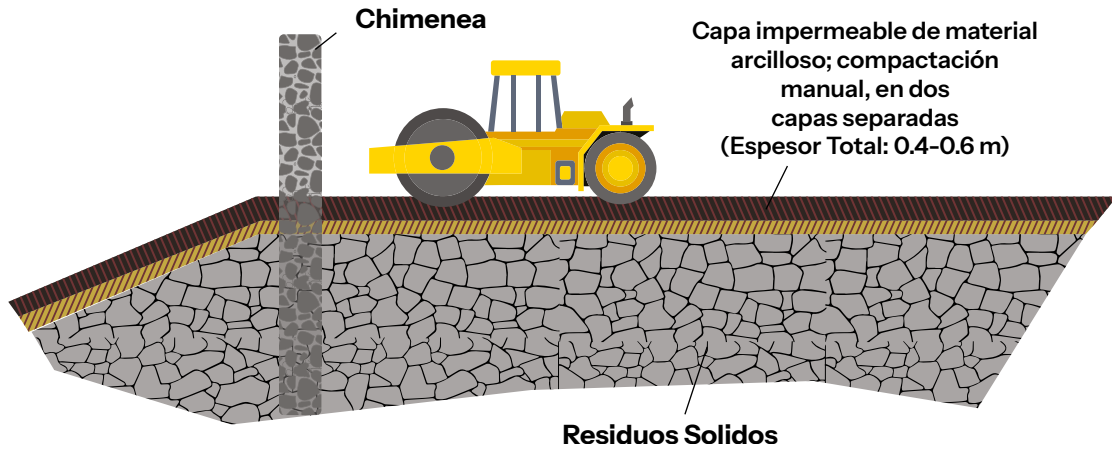
Figura 61. Construcción de capa impermeable.
