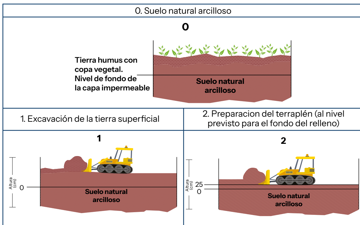
Figura 33. Construcción de capa base CON barrera natural.
