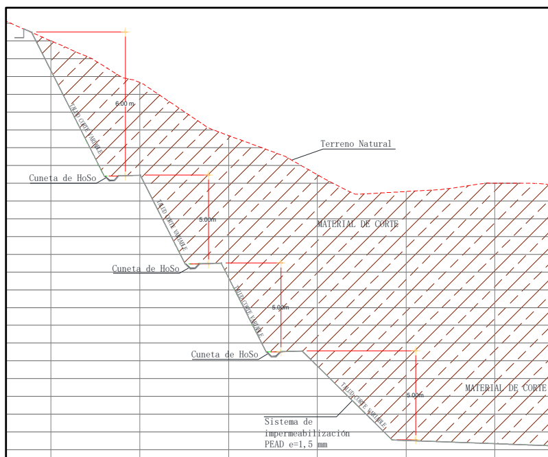
Figura 31. Imagen Esquemática de corte talud-banquina para emplazamiento en terrenos ondulados
