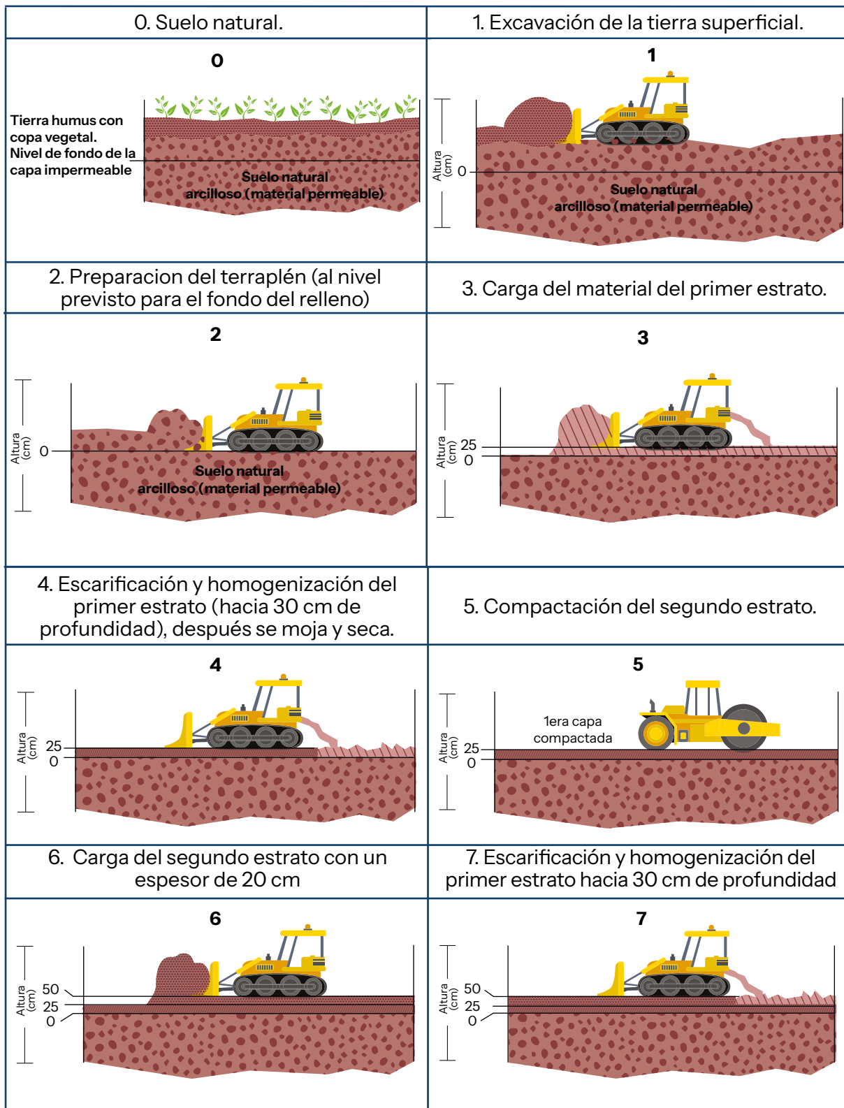
Figura 34. Construcción de capa base SIN barrera natural.
