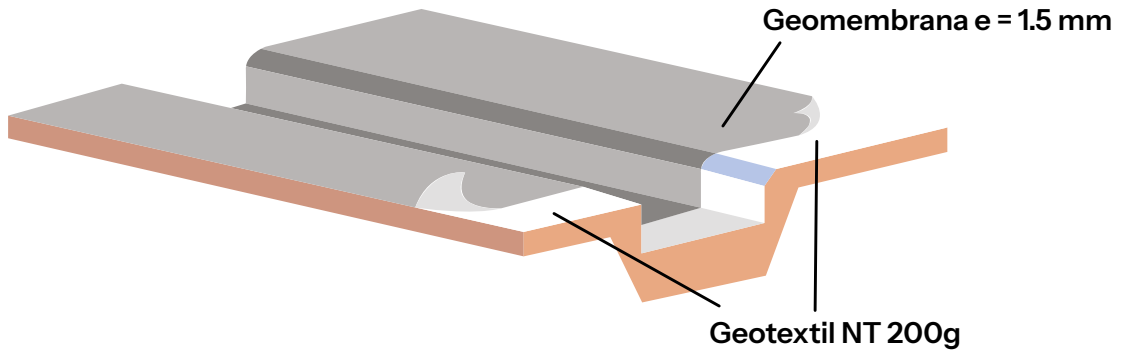
Figura 35. Sistema de impermeabilización sintética.
